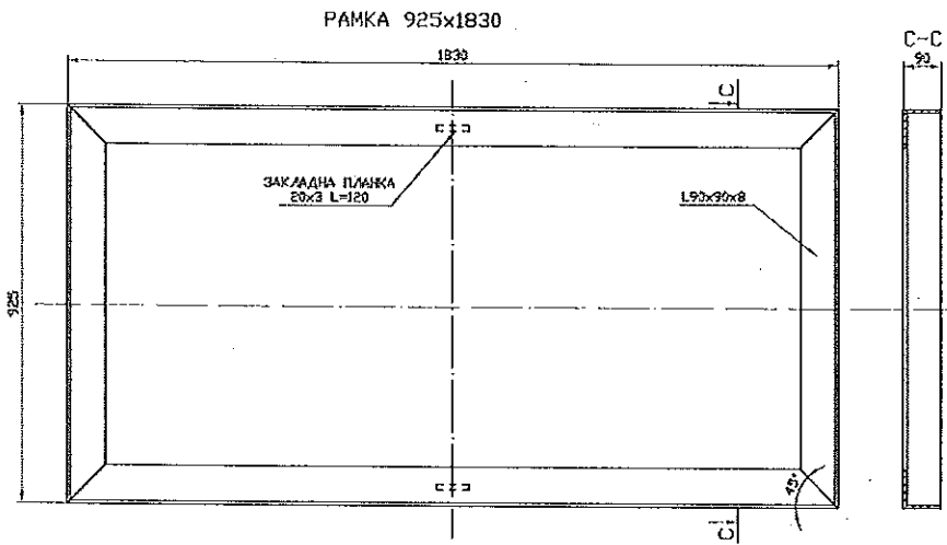
Фиг. 1 – Размери на метални рамки за капаци за кабелни шахти
