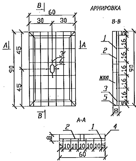
Фиг. 1. Кабелна шахта – единична ДЕТАЙЛ НА КАПАК ЗА ШАХТА 60/90
