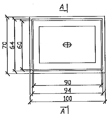
ДЕТАЙЛ - ШАХТА 60/90
