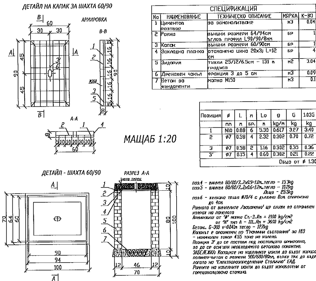
Фиг.6.3. Кабелна шахта – единична
