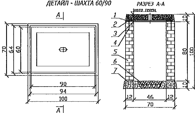
ДЕТАЙЛ - ШАХТА 60/90
