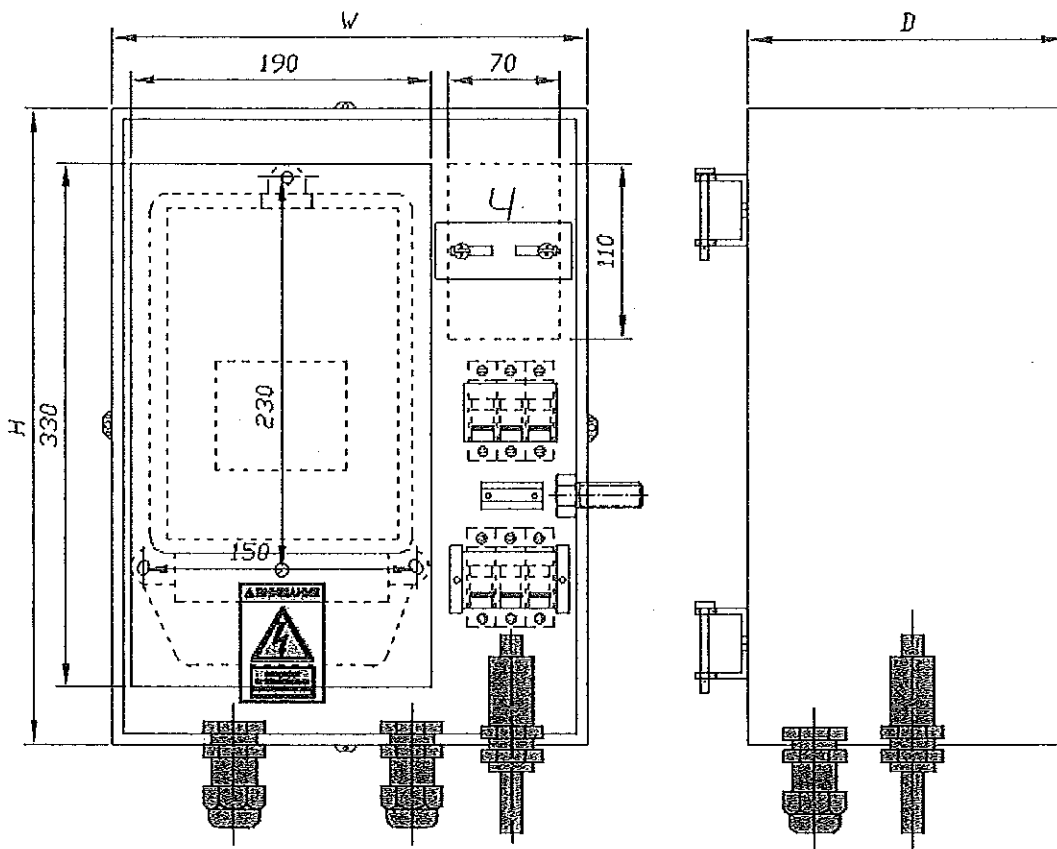
Фигура 4 – Електромерно табло 1-ПК-3Ф Основни размери и позициониране
