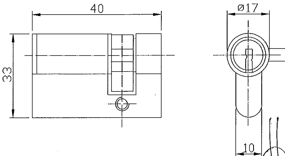
Фигура 1 - Патрон халф цилиндър със секрет
