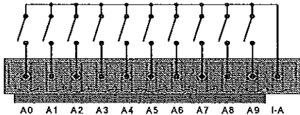
Рис. 39 – Активни DI
