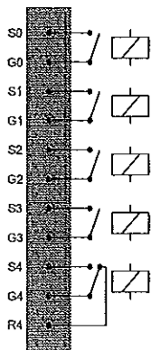
Рис. 37 – Конектор WAGO 231-541/001-000
