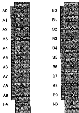
Рис. 41 – WAGO конектори
