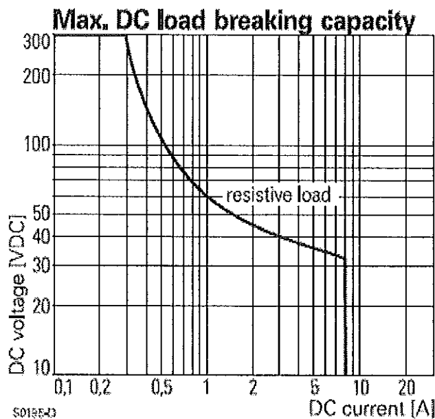
Рис. 36 – Характеристика на натоварванията на контактните релета
