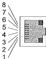
Рис. 34 - RJ45 конектор
