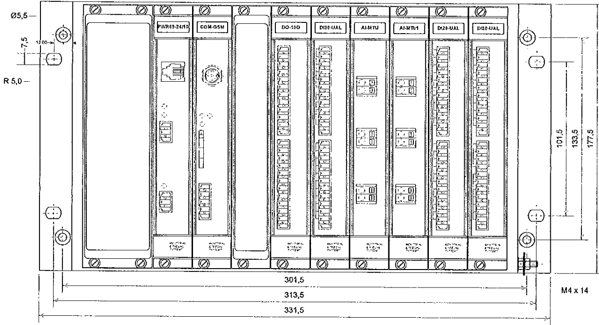
Рис. 7 – Размери на вана RTU7M-10
