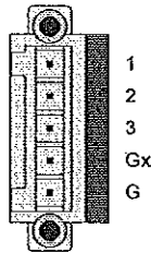
Рис. 56 - Конектор M3ZQ-BI
