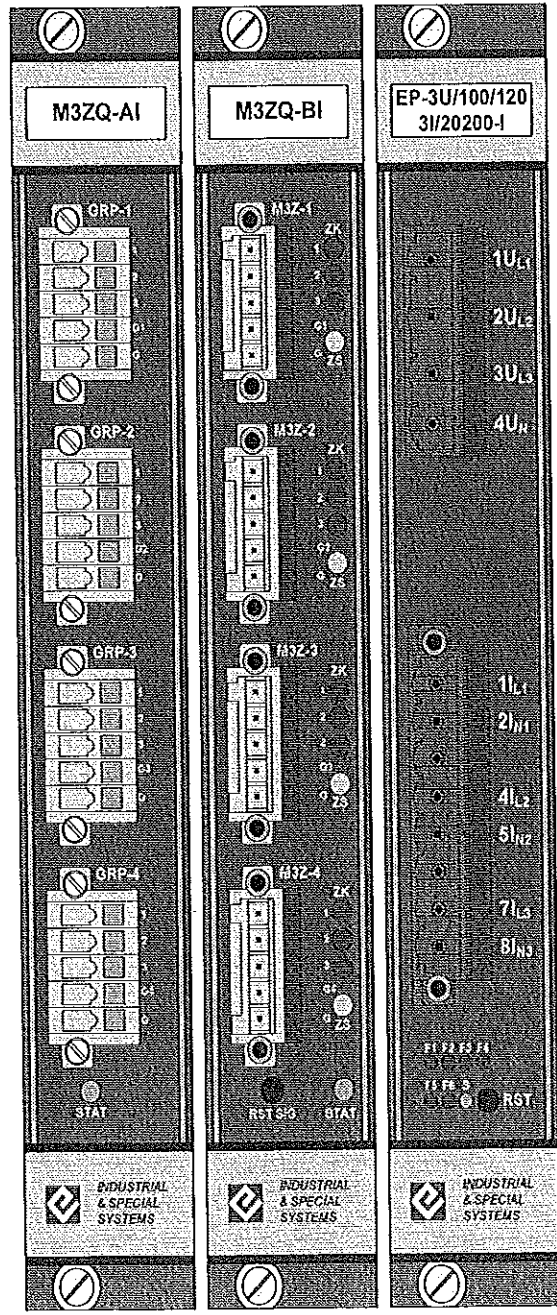
Puc. 61 - RTU7M-M3ZQ-AI, RTU7M-M3ZQ-BI, RTU7M-EP
