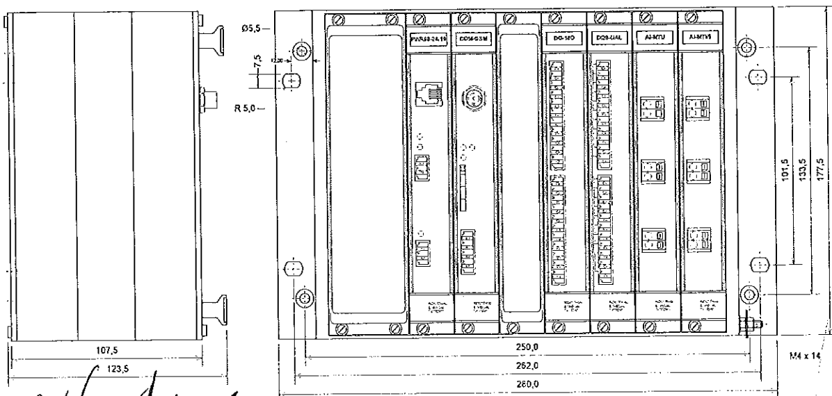
Рис. 6 – Размери на вана RTU7M-8
