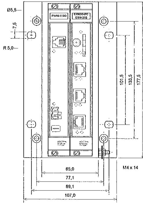
Рис. 4 – Размери на вана RTU7M-2
