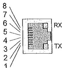
Рис. 21 – RS-232/RS-485
