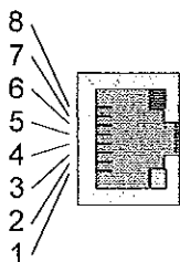
Рис. 17- NET конектор
