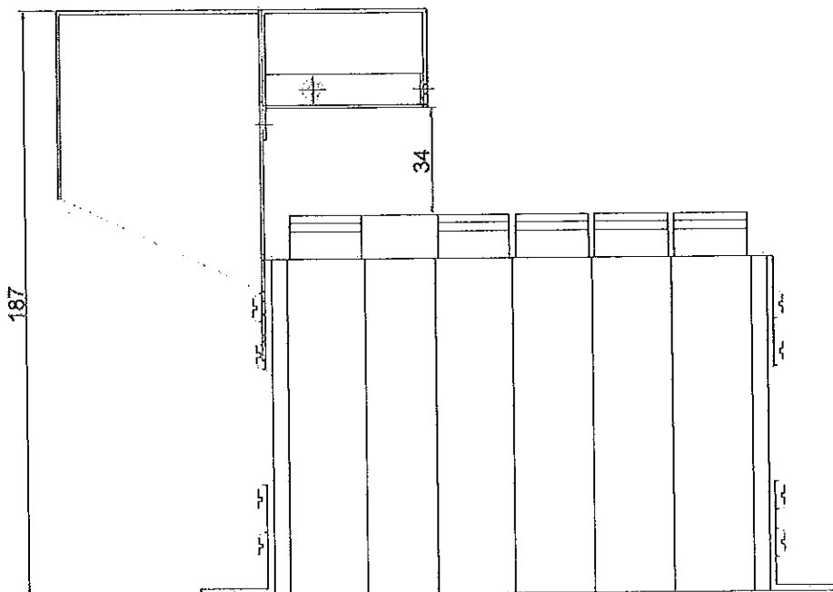
Рис. 10 - RTU7M-5 със сигнализация, поглед отдолу
