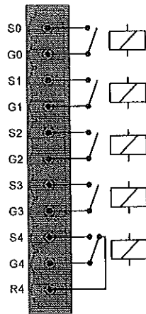
Рис. 46 – Конектор с дигитални изходи
