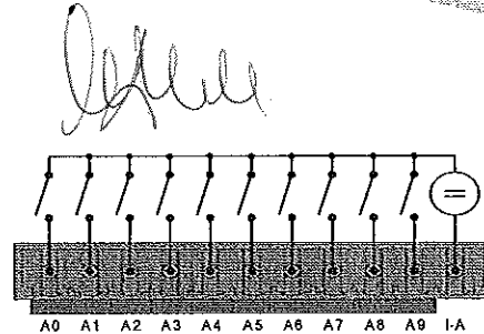
Рис. 40 – Пасивни DI
