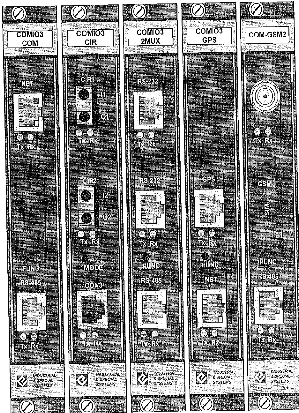
Рис. 19 – Поглед към челната част на модулите за връзка
