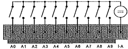
Рис. 44 – Пасивни DI
