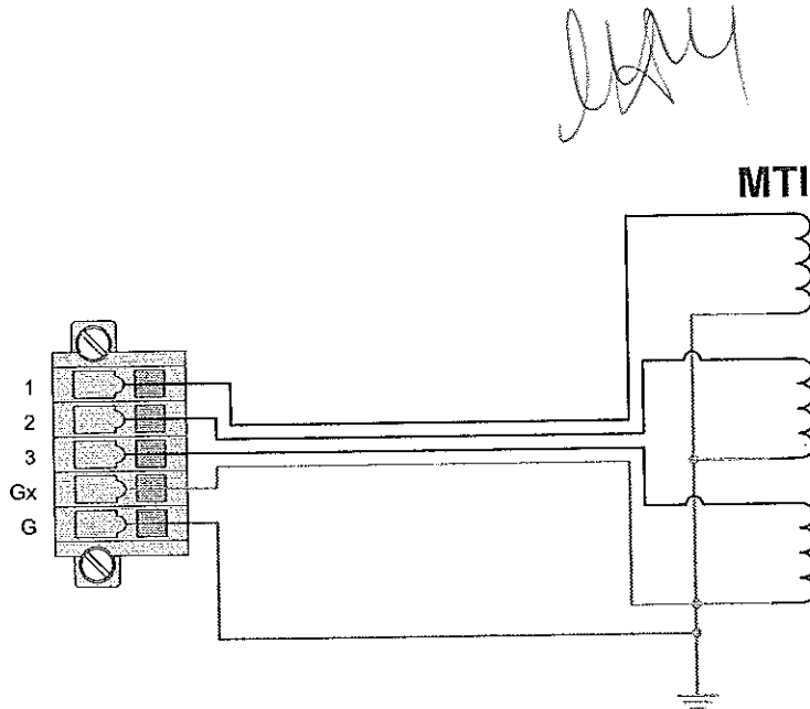
Рис. 53 – Свързване на аналоговите входове M3ZQ
