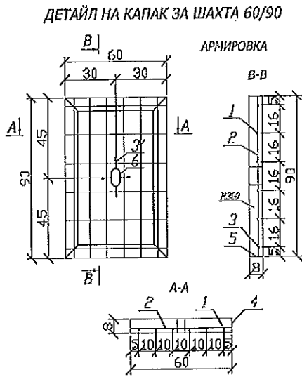
Фиг.7.3. Кабелна шахта – единична
