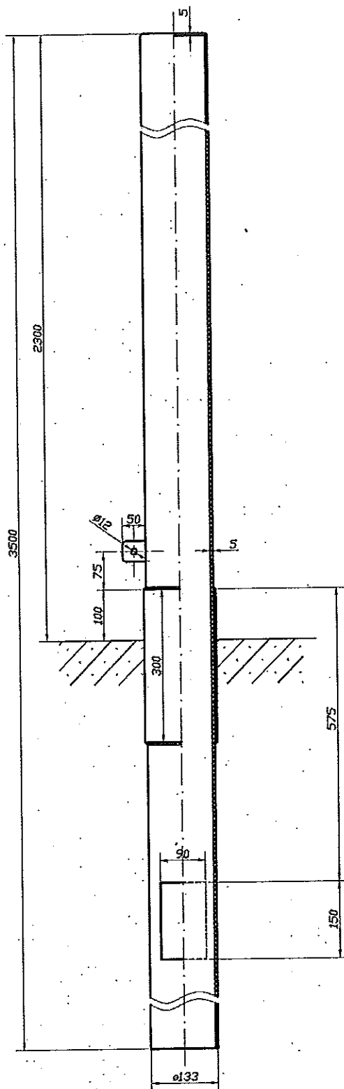
Фиг. 2 – Стоманотръбен стълб НН, безшевен – 3500/5 mm
