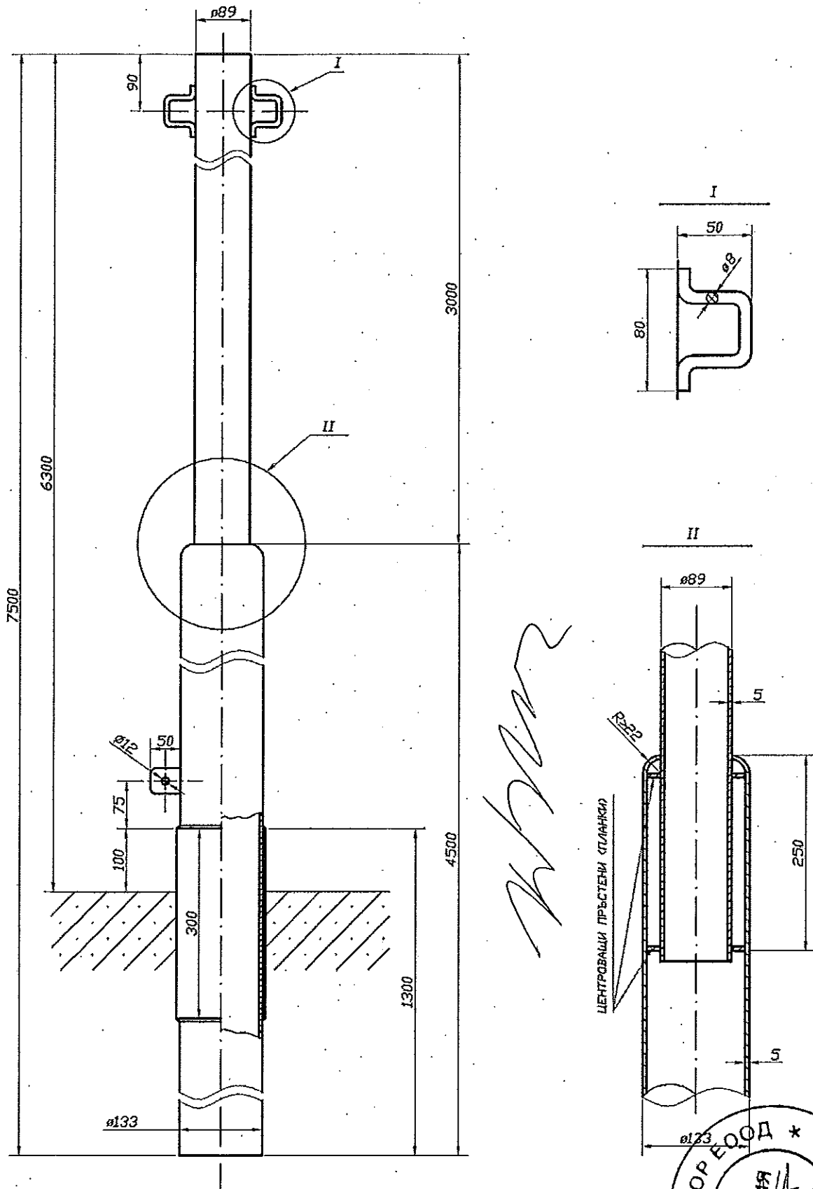
Фиг. 1 – Станотръбен стълб НН, безшевен, 7500/5 mm - 111кв.
