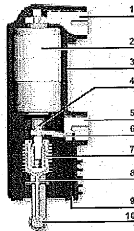
Вакуумна дългогасителна камера, вградена в епоксиден полюс
